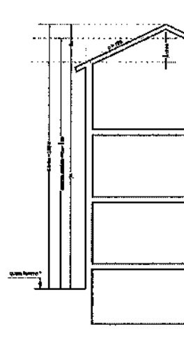
Figura 3 (Art. 94, comma 1, punto c) Edifici con coperture a falde con pendenza superiore al 32%: l'altezza va misurata sommando alla altezza ottenuta, come al punto precedente, l'1/20 dell'altezza sino al colmo del tetto, calcolata dal punto di congiunzione tra la verticale esterna del muro perimetrale e l'introdosso della falda di copertura. Il valore in ogni caso non potrà essere superiore a m. 3,00 dall'altezza massima consentita per l'edificio.
